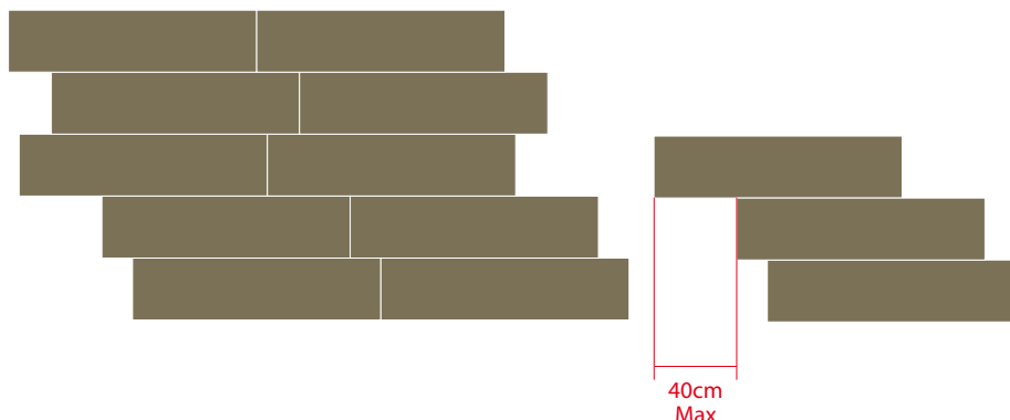
4 - Укладка вразбежку с хаотичным смещением 4 - Posa a modulo irregolare 4 - Irregular module installation pattern
